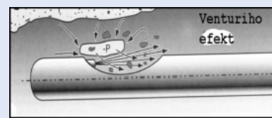
Obrázek 9. Princip Venturiho efektu Hydrolyzeru
